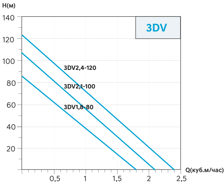
рисунок 1. График напорных характеристик
