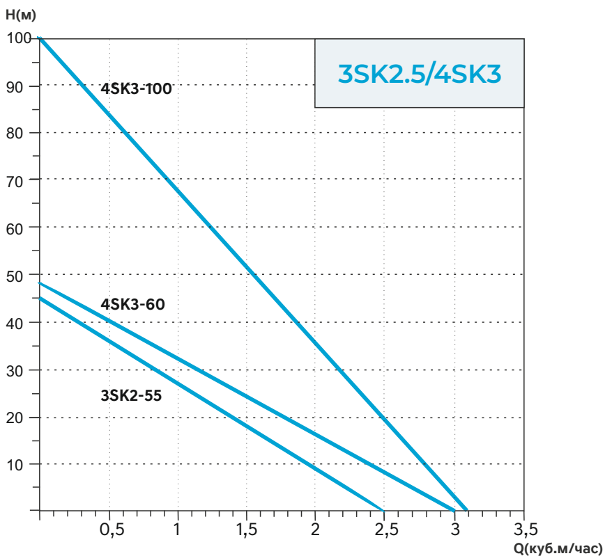
рисунок 1. График напорных характеристик
